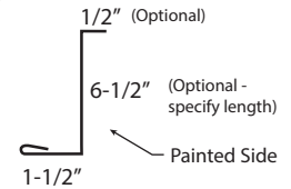
㉒ Fascia Trim
